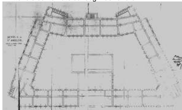
Pianta del primo piano nel progetto originale
