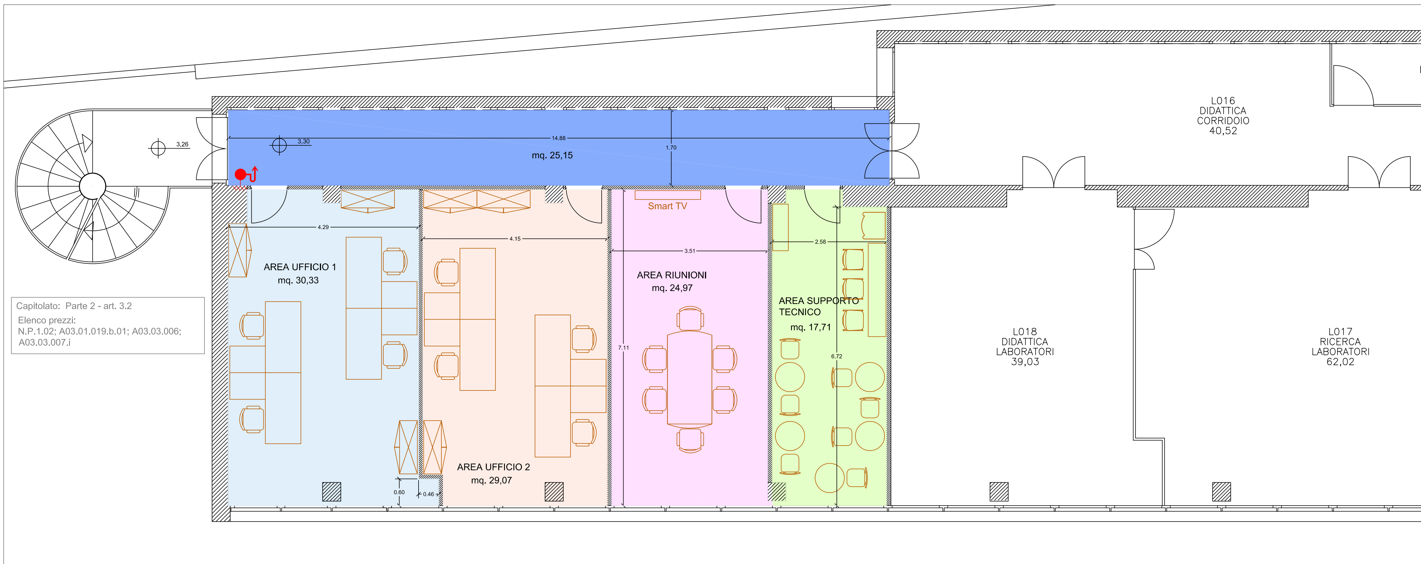
Pianta arredata - Piano primo
