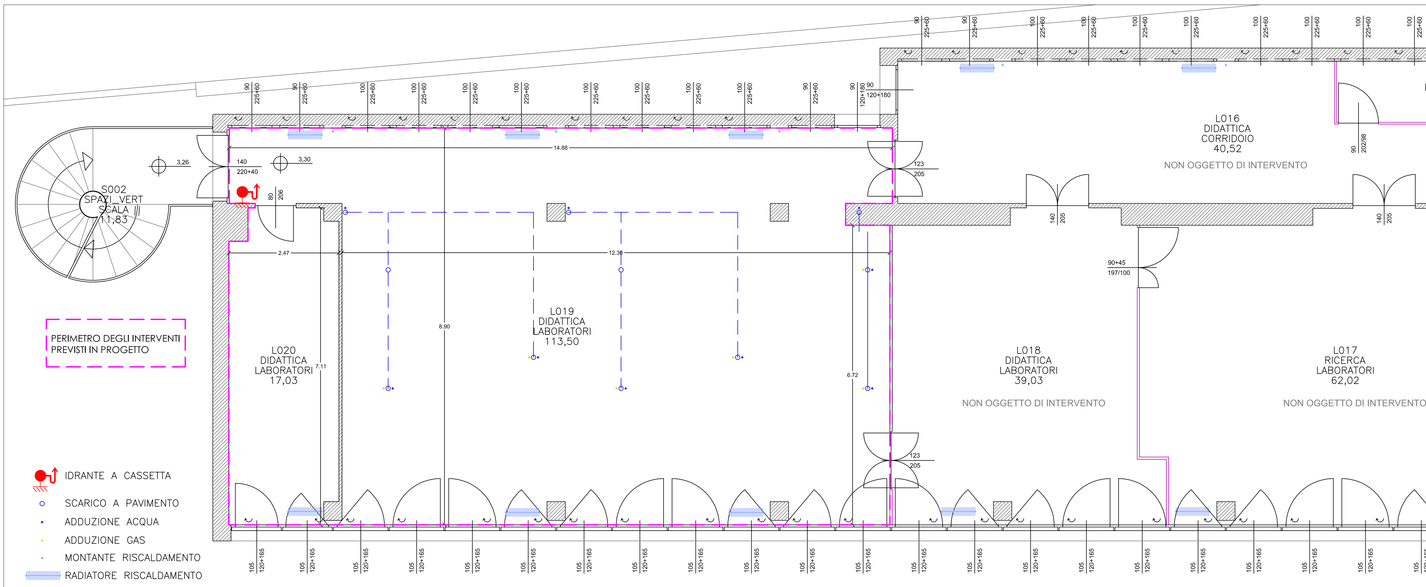
Pianta Stato di fatto - Piano primo
