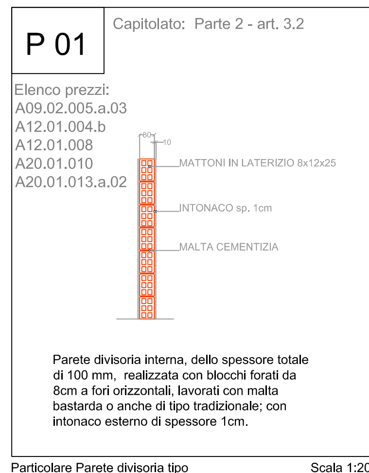
Scala 1:20
