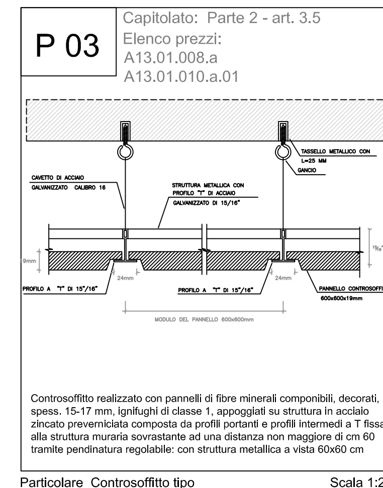
Scala 1:20
