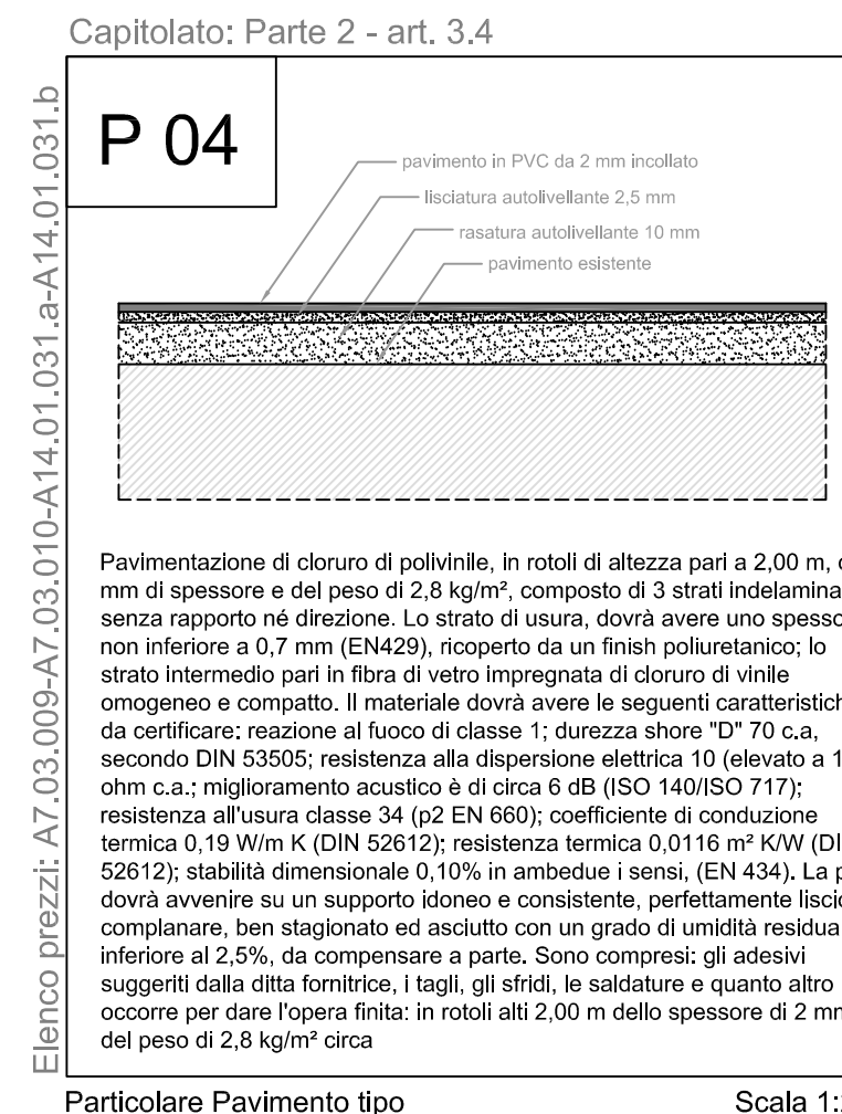
Scala 1:20
