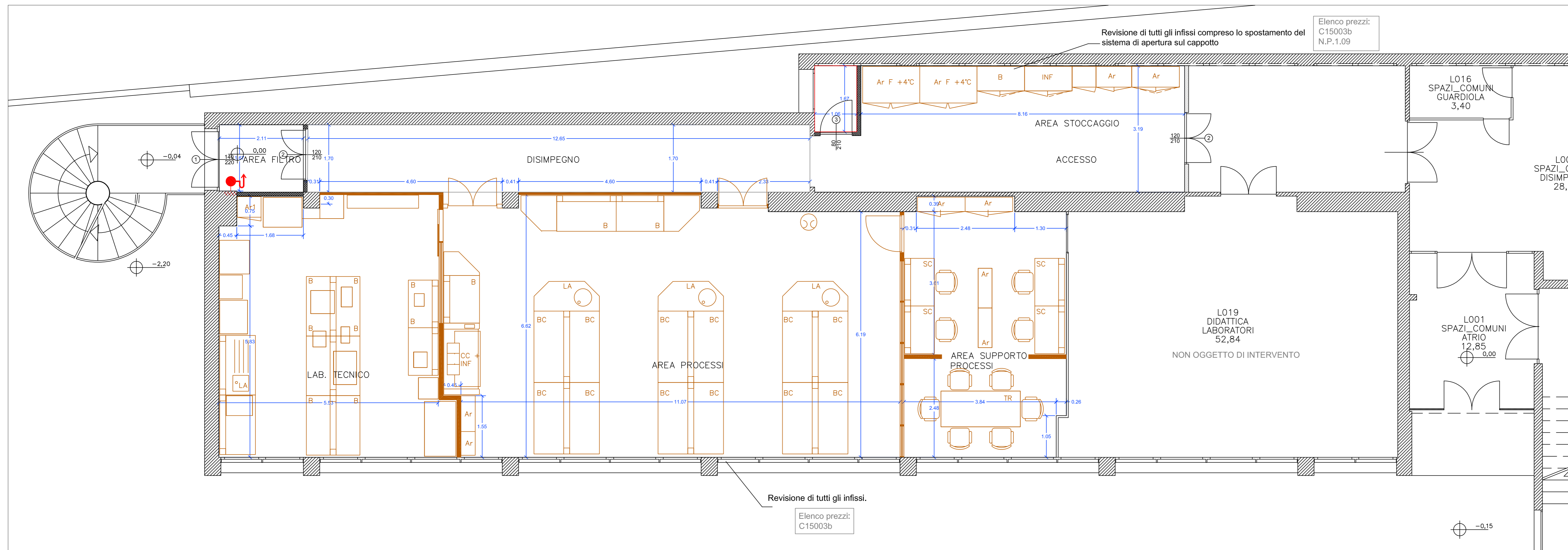
Pianta Stato di Progetto - Piano terra SCALA 1:50
