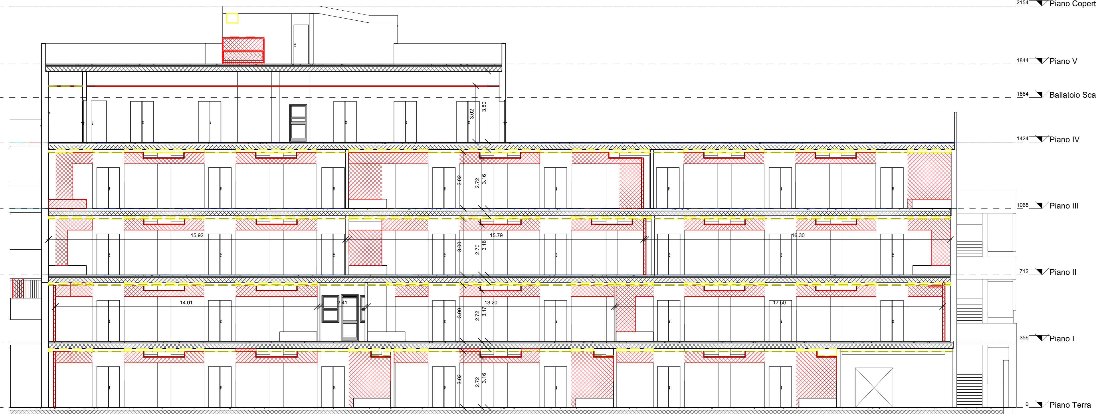
SEZIONE COMPARATIVA 2 DEMOLIZIONI-RICOSTRUZIONE
