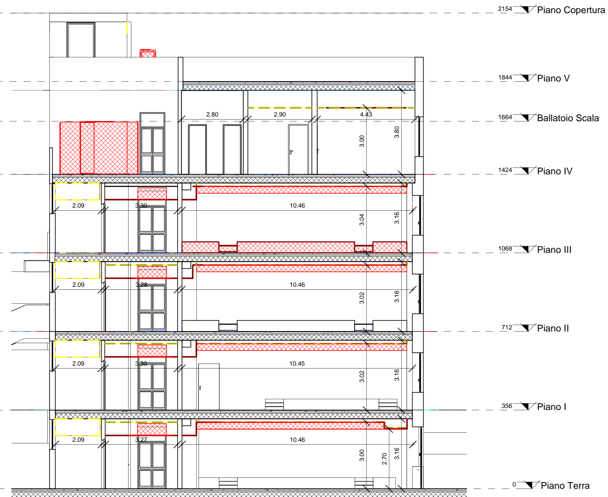
SEZIONE COMPARATIVA 3 DEMOLIZIONI-RICOSTRUZIONE
