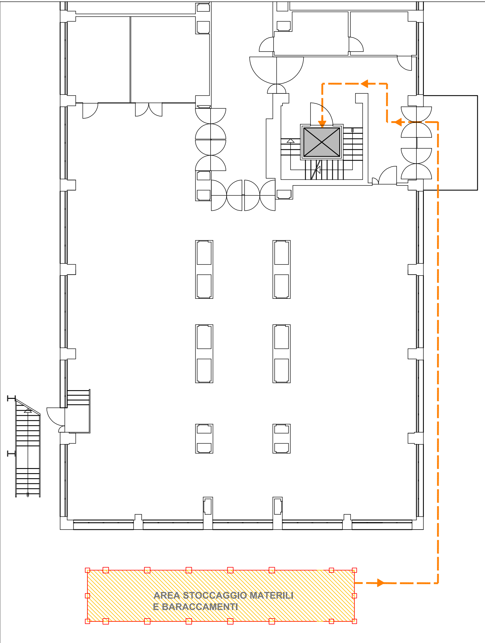
PLANIMETRIA AREA DI CANTIERE QUOTA STRADA
