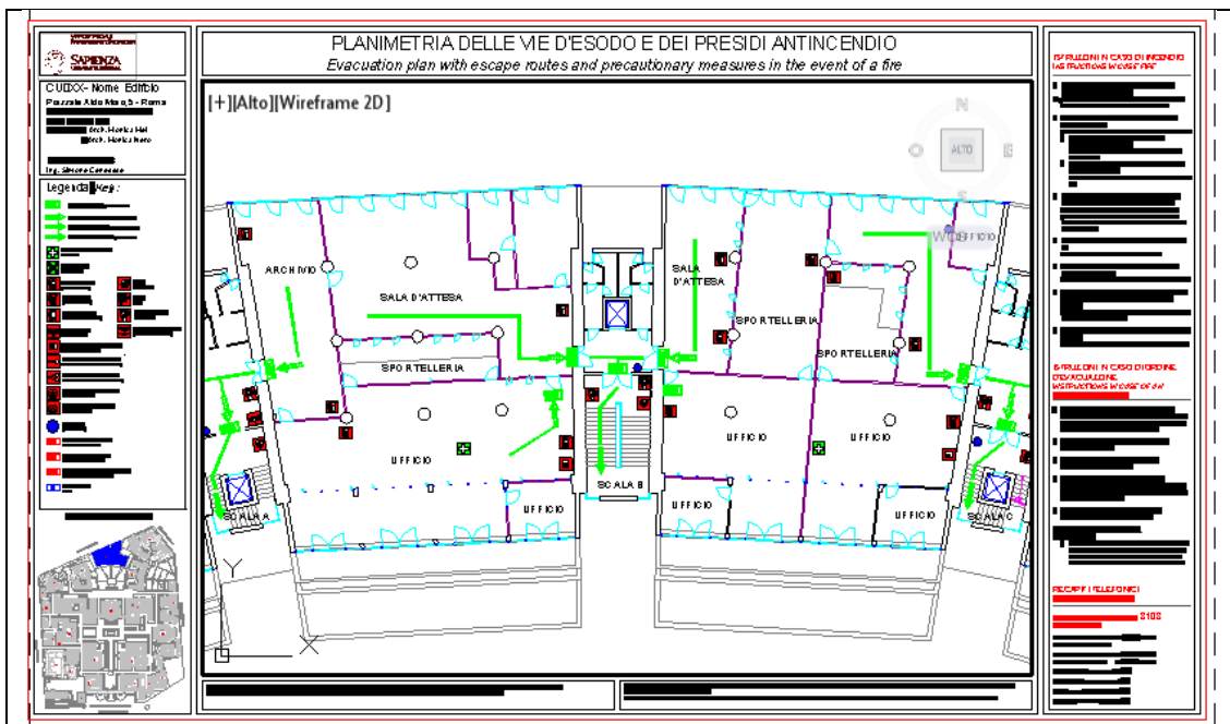
Fig. 1 – Esempio di Planimetria riportante le Vie di Fuga
