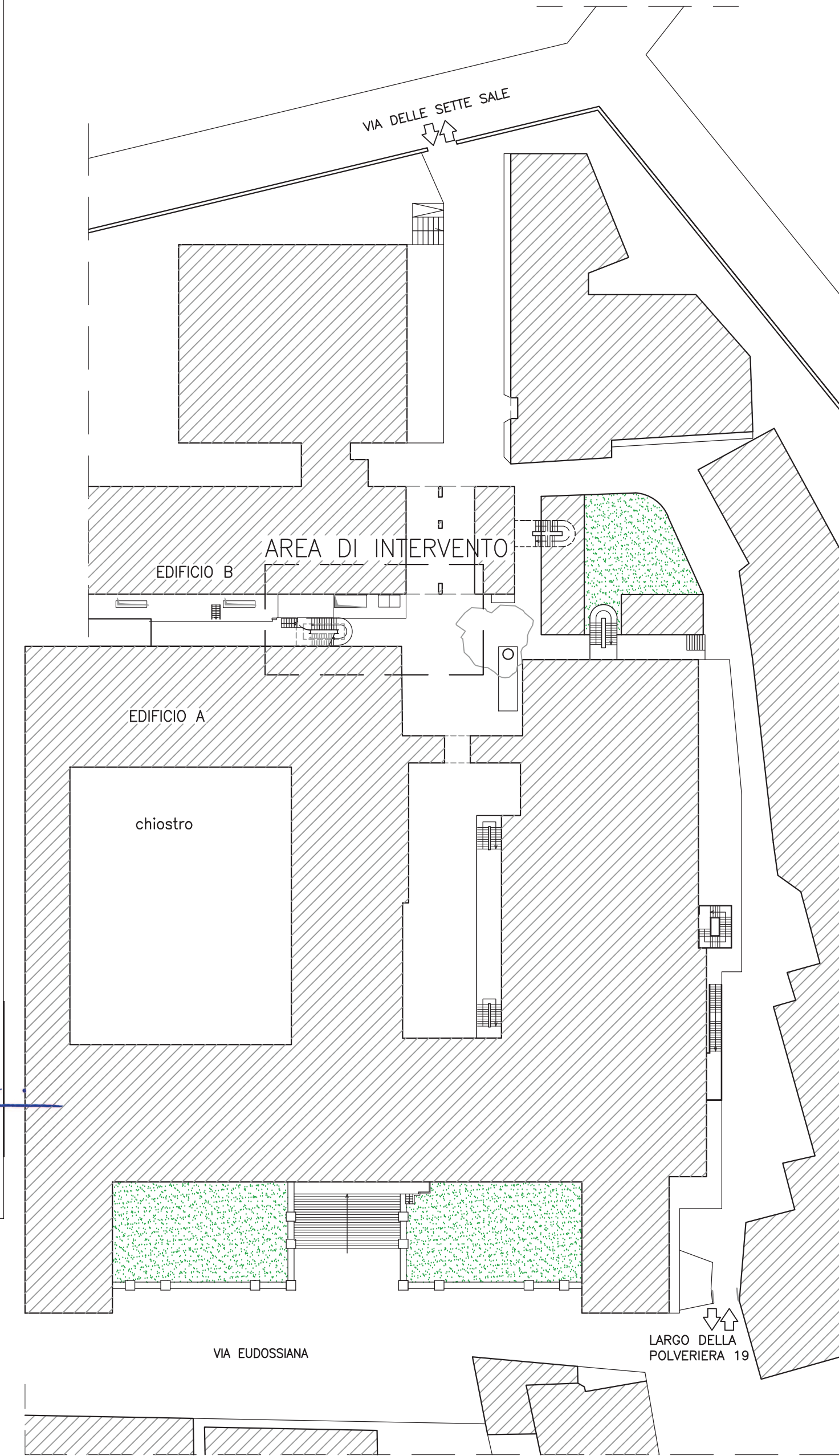
Planimetria generale Scala 1:500
