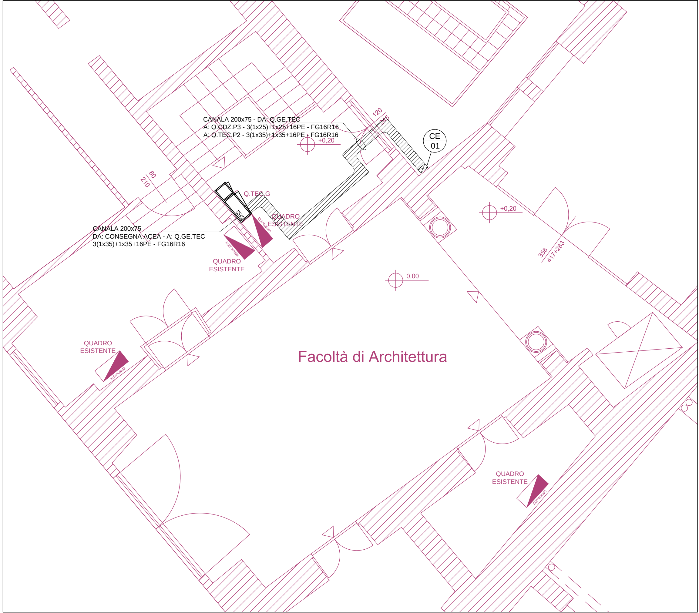
STRALCIO Pianta Piano Terra - Scala 1:50
