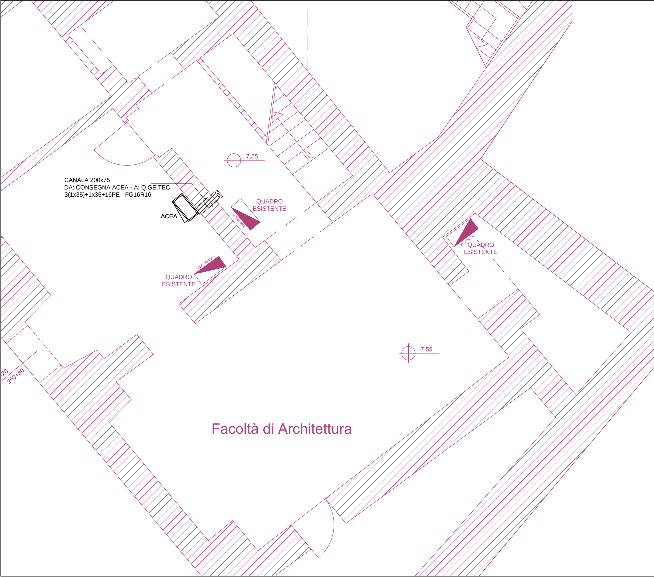
STRALCIO Pianta Piano Interrato - Scala 1:50
