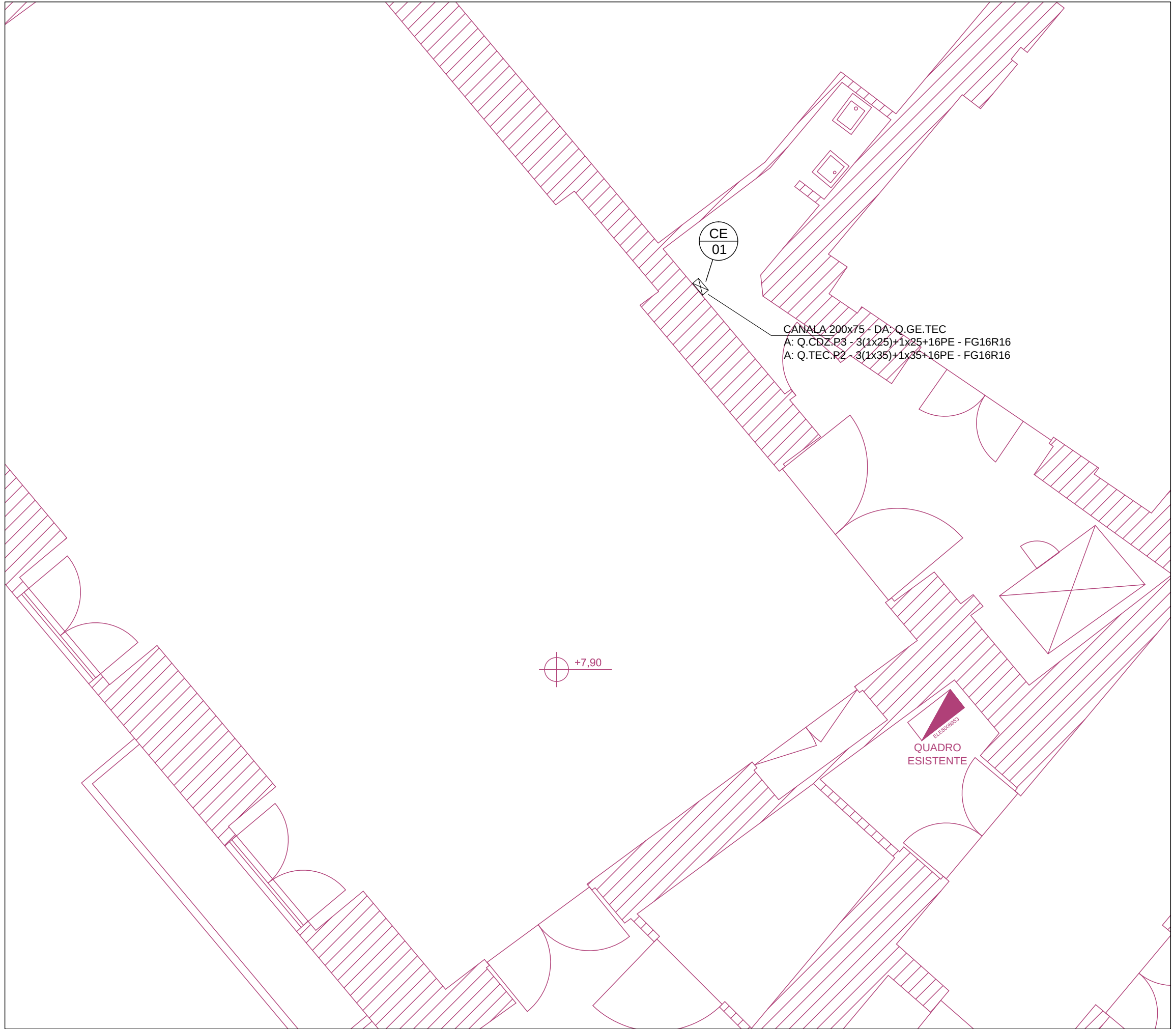
STRALCIO Pianta Piano Primo - Scala 1:50
