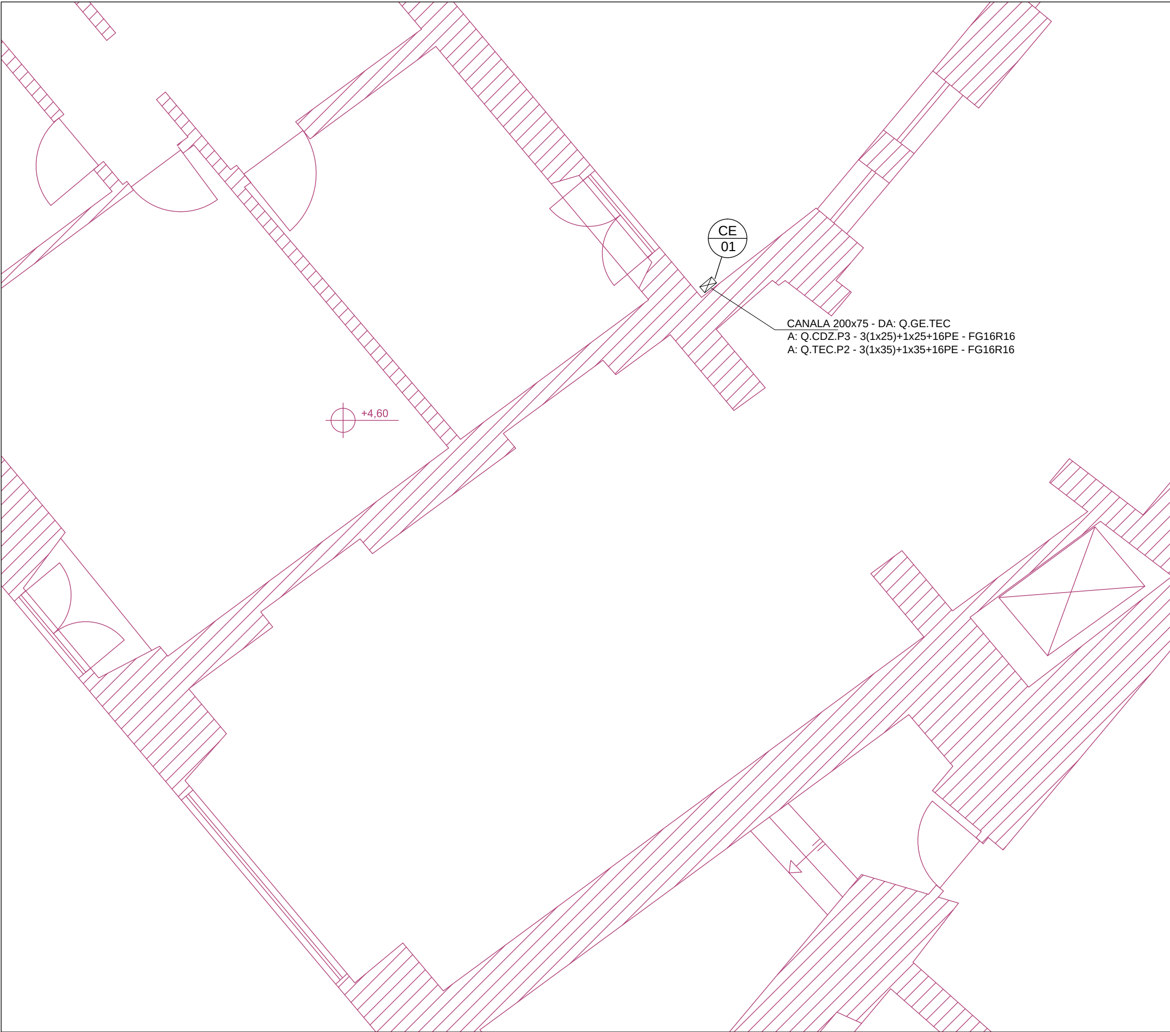
STRALCIO Pianta Piano Ammezzato Terra - Scala 1:50
