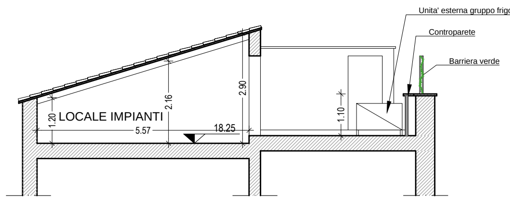
SEZIONE E-E'
