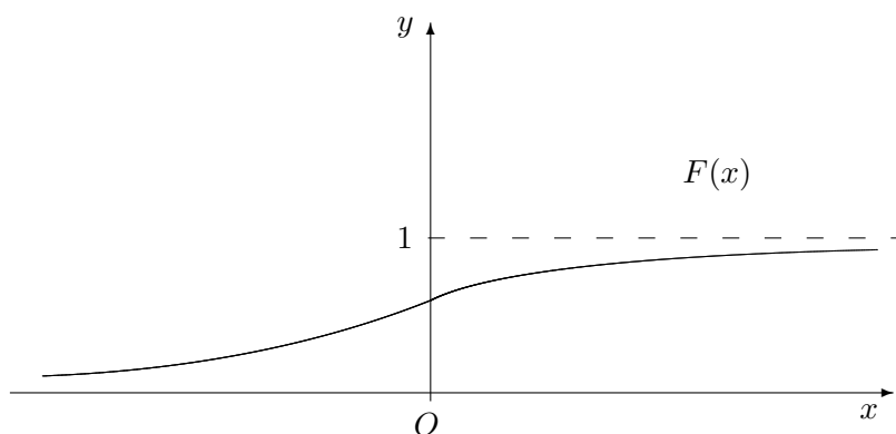
Figura 1. Tipico grafico di una funzione di ripartizione di una v.a. continua
