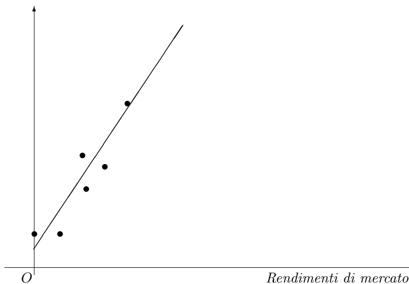
Figura 16. Retta di regressione con \alpha = 1,955 , \beta = 1,448
