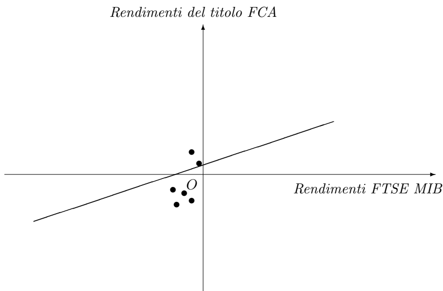
Figura 17. Retta di regressione per FCA con \alpha_{FCA} = 0,003 , \beta_{FCA} = 0,3
