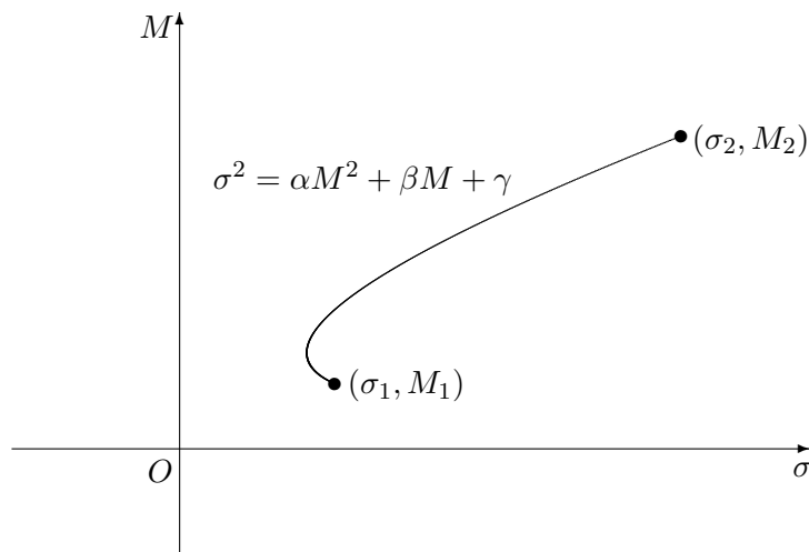
Figura 5. Ramo di iperbole nel piano Rischio-Rendimento
