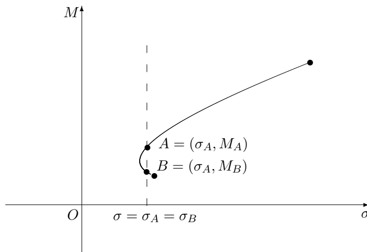
Figura 8. A parità di volatilità, A è preferito a B nel ramo di iperbole
