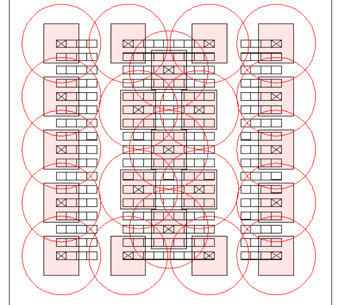
Schema con distanziamento 2.25 m
