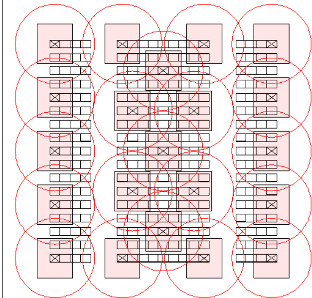
Schema con distanziamento 2.25 m
