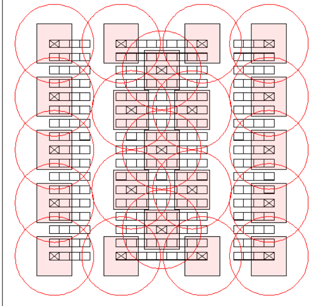
Schema con distanziamento 2.25 m
